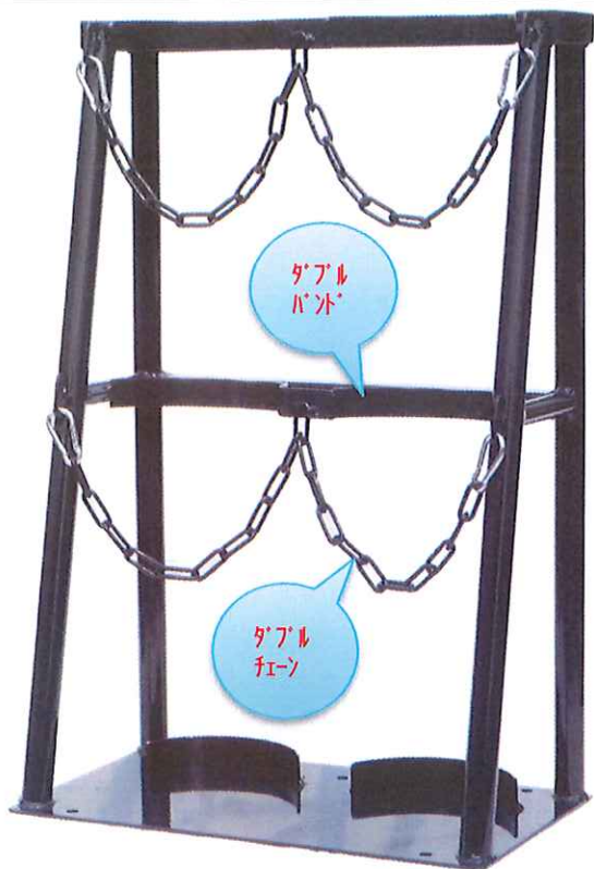
■ ボンベスタンド1500ℓ × 2本立上中バンド仕様
