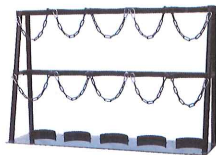
■ ボンベスタンド1500ℓ × 5本立上中バンド仕様
