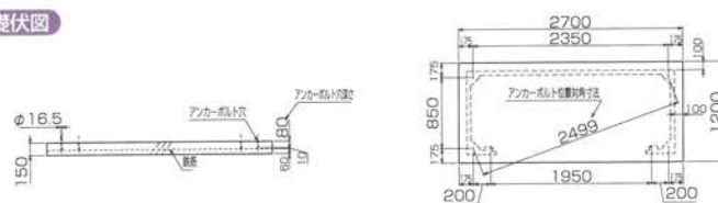
基礎伏図
