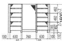
正面図
