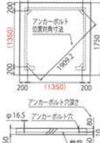
基礎図
