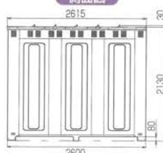
側面図
