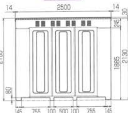
背面図
