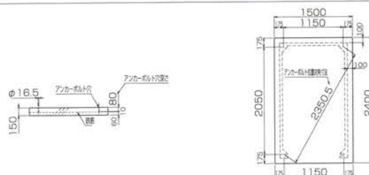
基礎伏図
