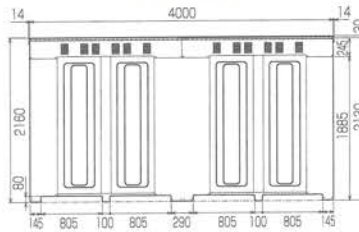
背面図
