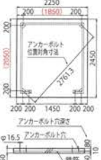
基礎図
