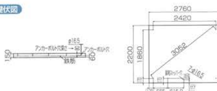
基礎伏図
