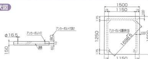
基礎伏図
