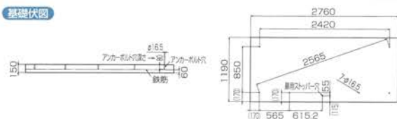
基礎図
