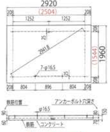
基礎伏図
