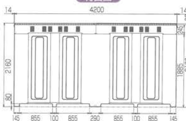
背面図
