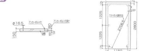
正面図
