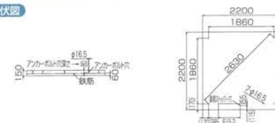
基礎伏図
