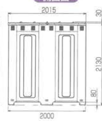
側面図
