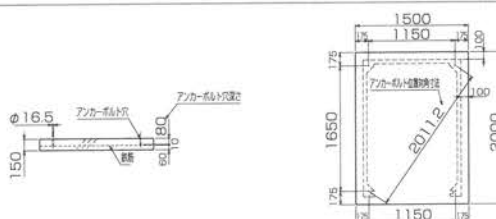
基礎伏図
