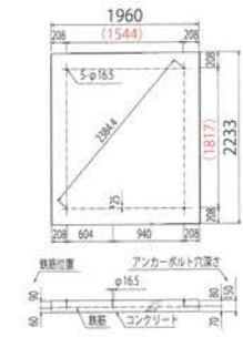
基礎伏図
