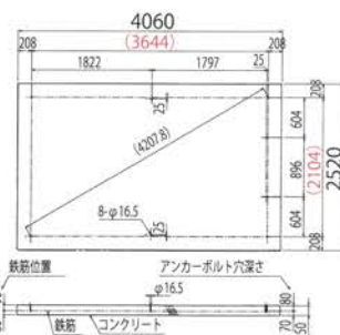
基礎伏図
