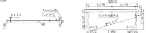
正面図
