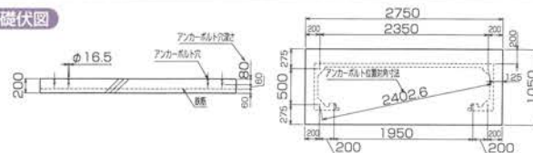
基礎伏図
