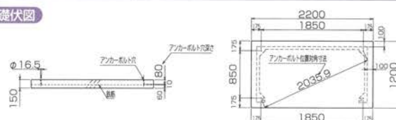
基礎伏図
