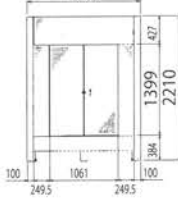
正面図
