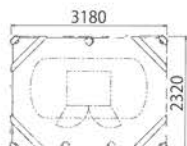
平面図
