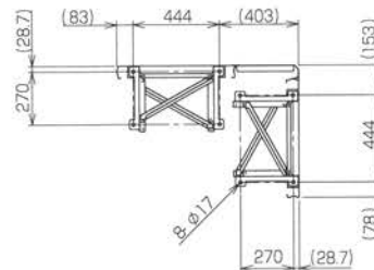
アンカー寸法
