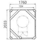
平面図
