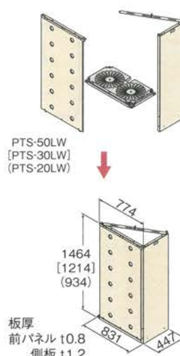
〈図面〉LW型
