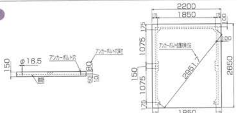
基礎伏図
