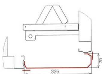
詳細図 A
