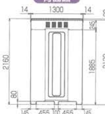
背面図
