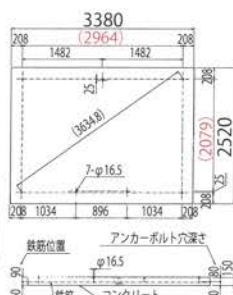
基礎伏図
