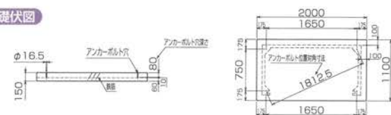
基礎伏図
