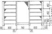
正面図
