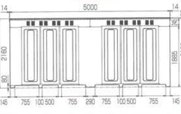
背面図
