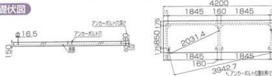
基礎伏図
