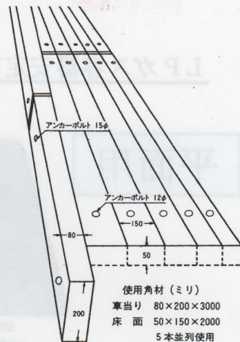
車当り 80×200×3000 容器卸場 50×150×2000 (並列 5 本)
